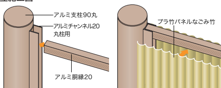
アルミ支柱90丸ブラウン
