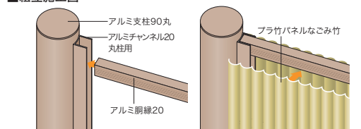
アルミ支柱90丸ブロンズ
