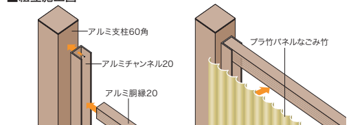
アルミ支柱60角ブロンズ
