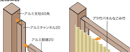
アルミ支柱60角ブラウン
