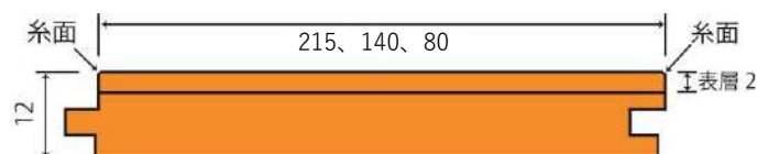
断面図 (表層2mm無垢挽き板) 本実式
