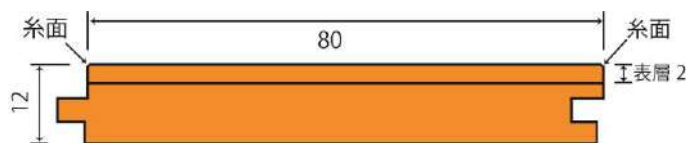
断面図（表層2mm無垢挽き板）本実式
