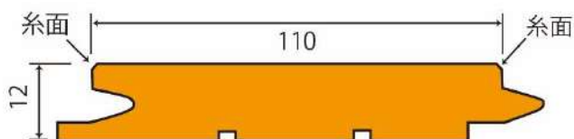
断面図 (12mm厚)
