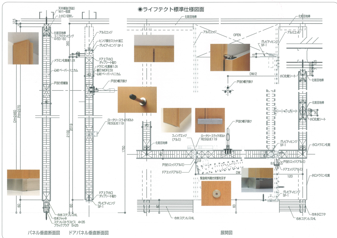
標準仕様例 MARRX-H
