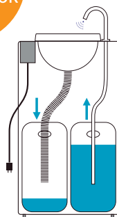
排水用 給水用 タンク タンク
