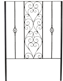
JHIF-V01 サイズ H1400×W1000×D30 重量 25kg
