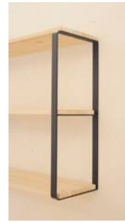
シェルフブラケットM MUK-1563 W270 D32 H700 ・サンドブラック塗装 ・クリア塗装 重量2.4kg/個 棚板別売り
