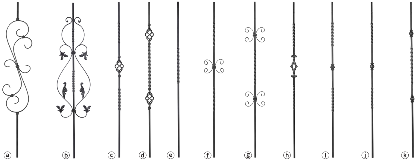
(a) JHIK-06 サイズ H1100×W210 ■14×14mm 重量 3.2kg (b) JHIK-07 サイズ H1100×W235 ■14×14mm 重量 3.3kg (c) JHIK-01 サイズ H1100×W70 ■14×14 重量 1.6kg
