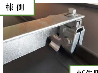
軒先側
