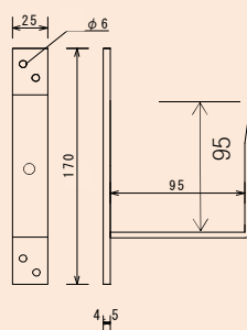
貫抜き 受け 90角用
