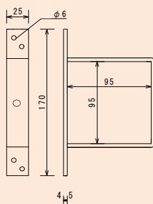
貫抜き 通し 90角用
