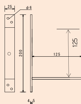
貫抜き 受け 120角用
