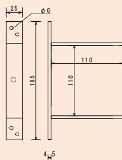
貫抜き 受け 105角用
