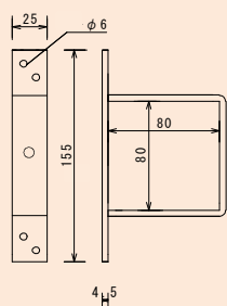
貫抜き 通し 75角用
